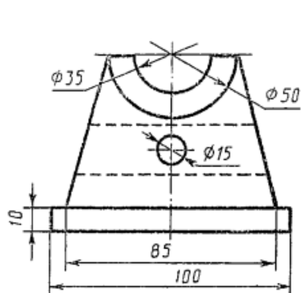
Стойка
