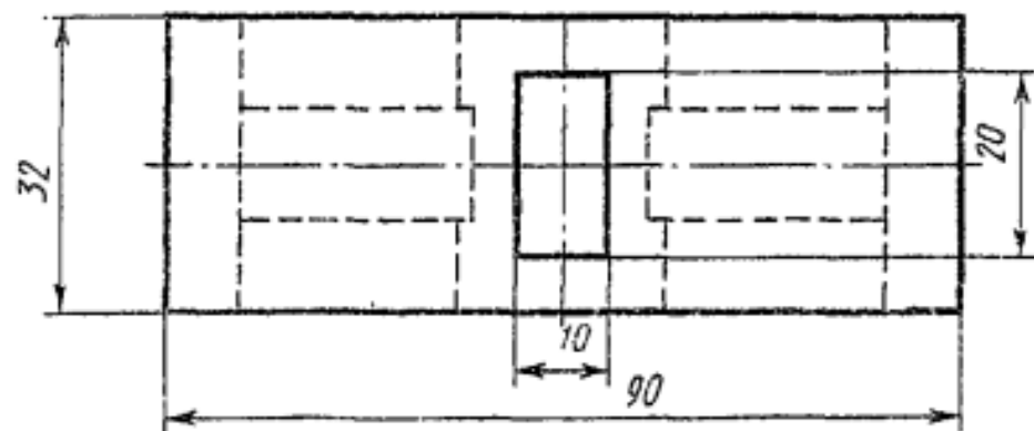
Призма
