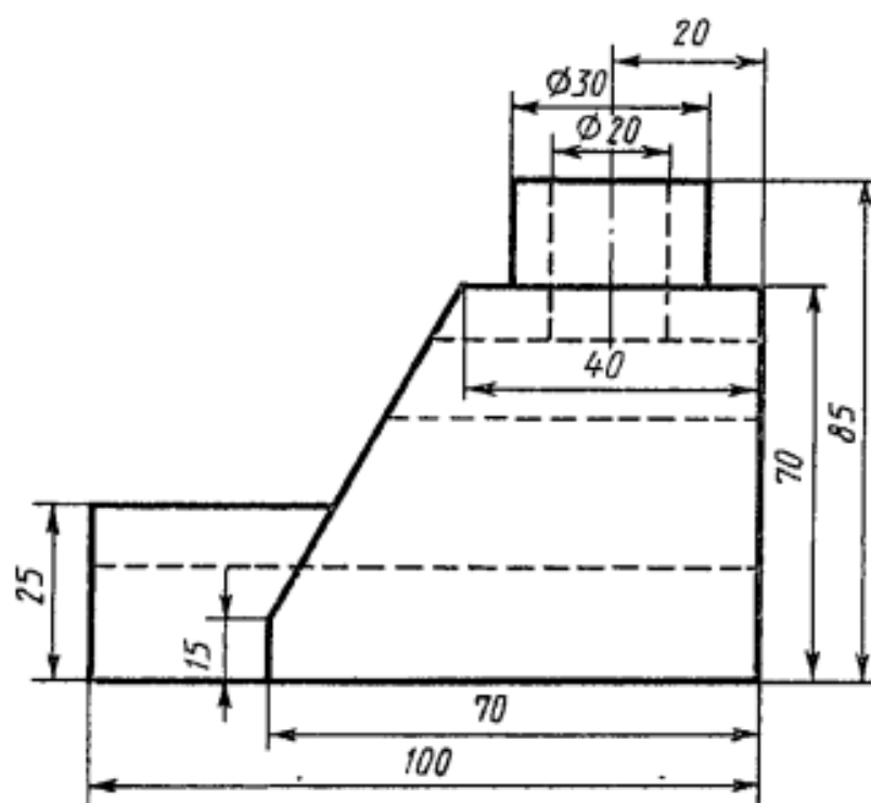
Стойка
