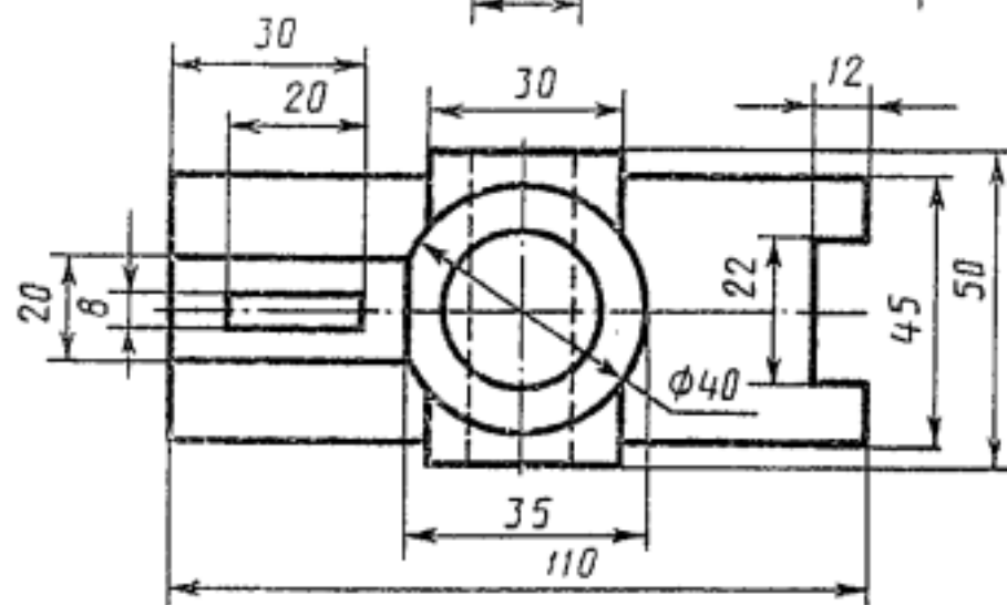
Корпус
