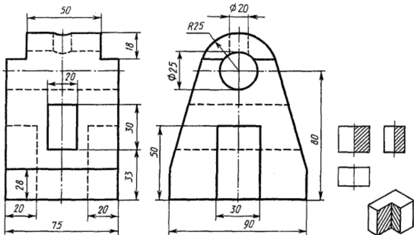
Стойка
