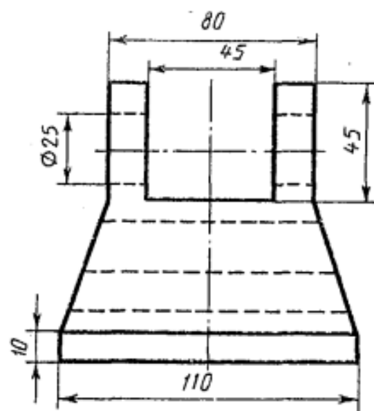
Опора
