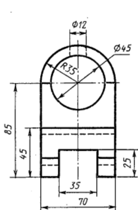
Кронштейн
