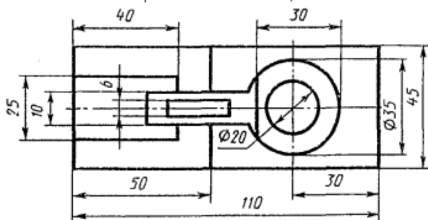
Вилка
