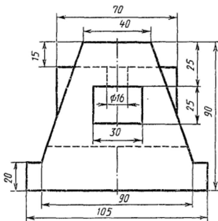
Станина
