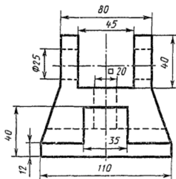
Кронштейн
