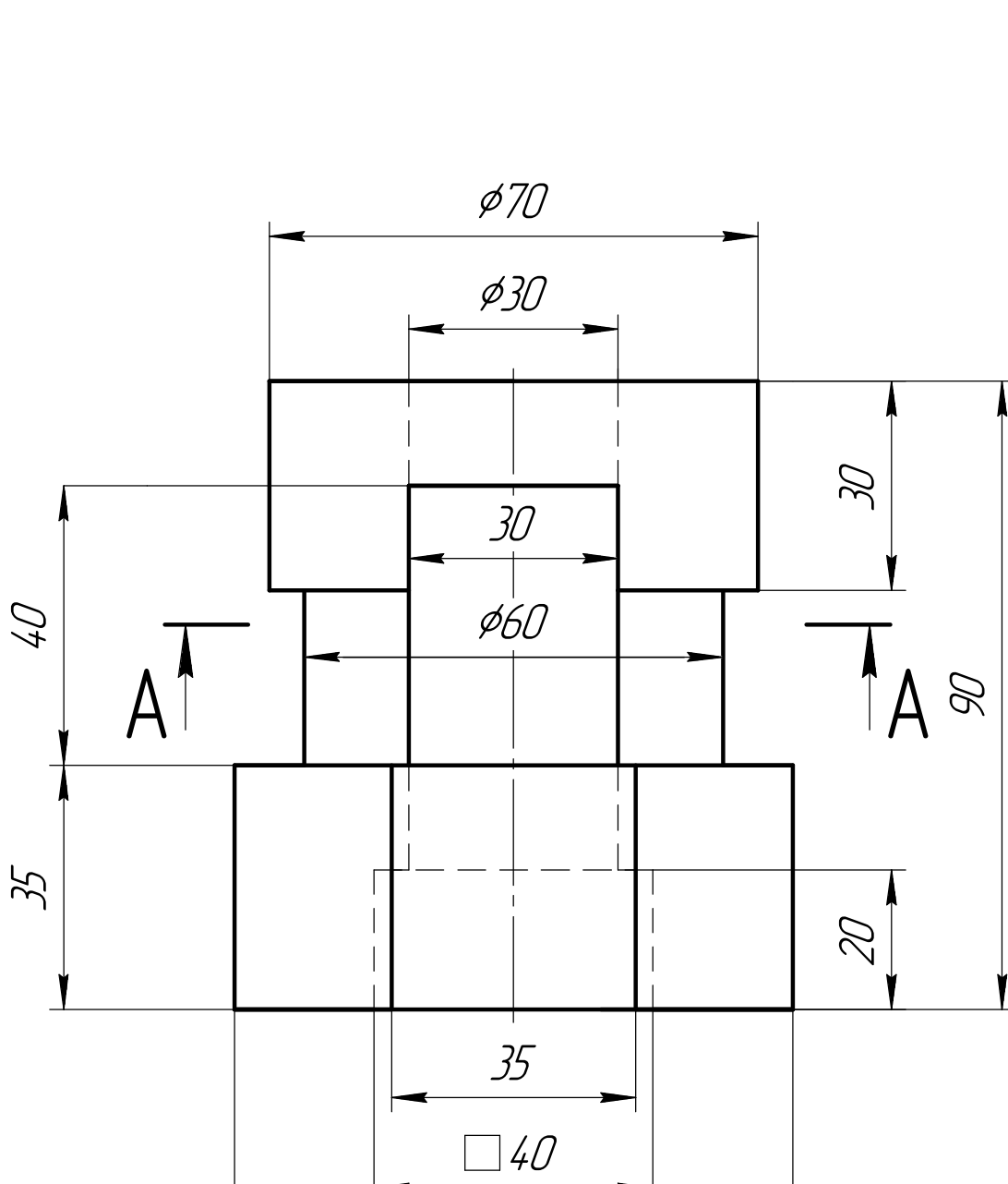
вариант 25 Вид спереди
