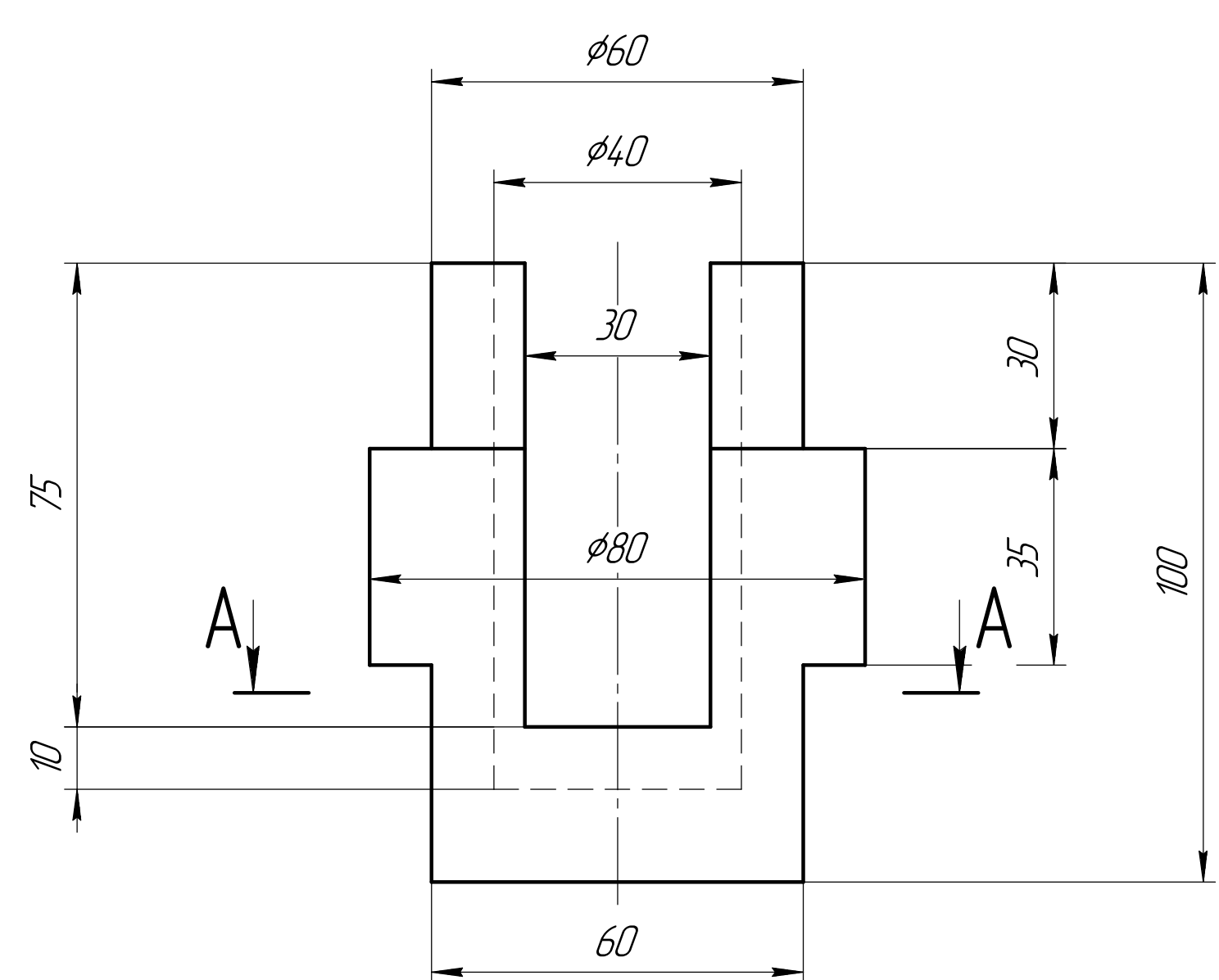
вариант 1 Вид спереди
