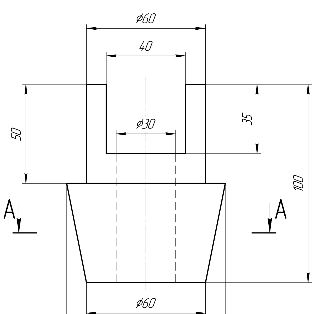
вариант 5 Вид спереди
