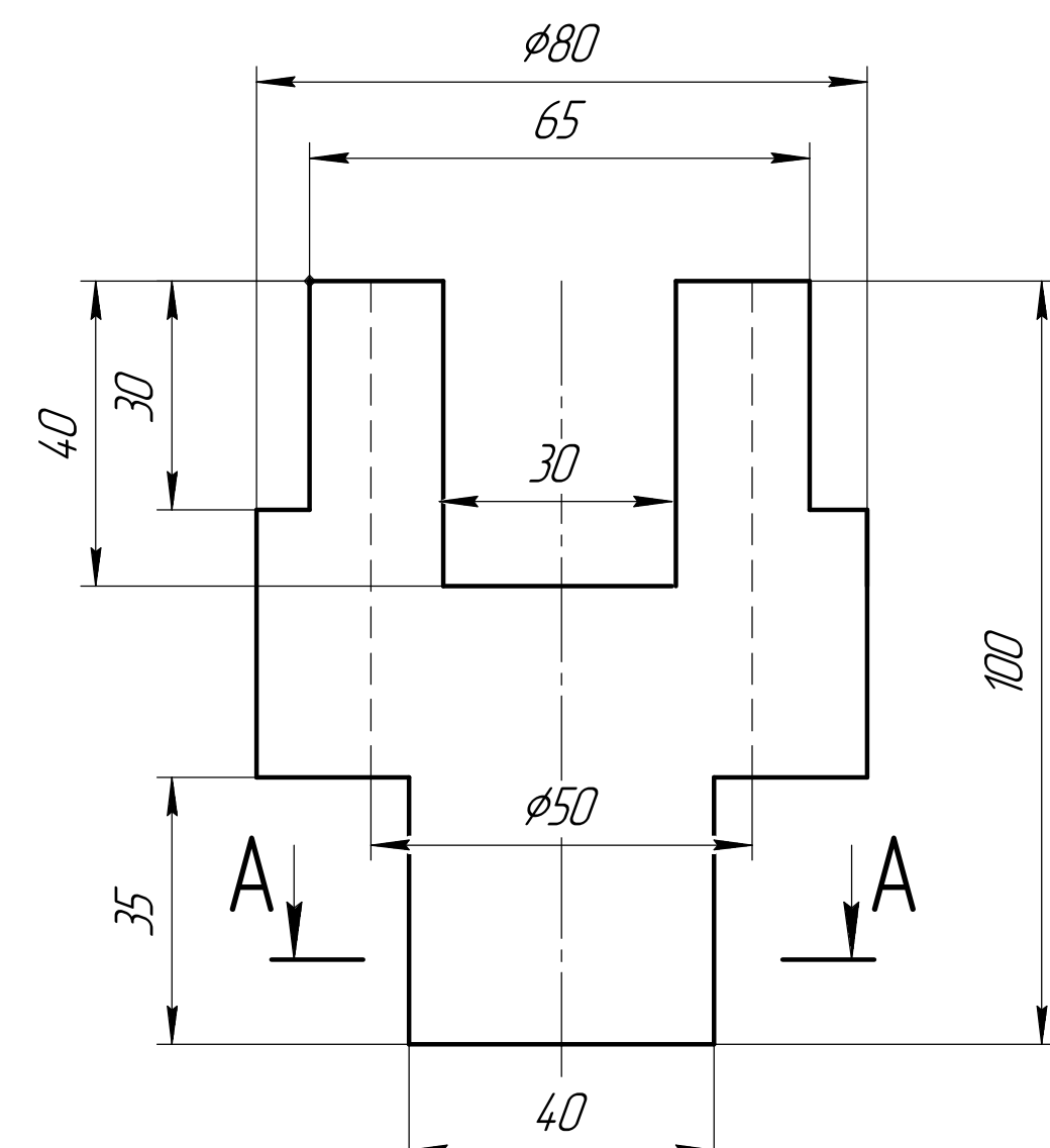
вариант 15 Вид спереди
