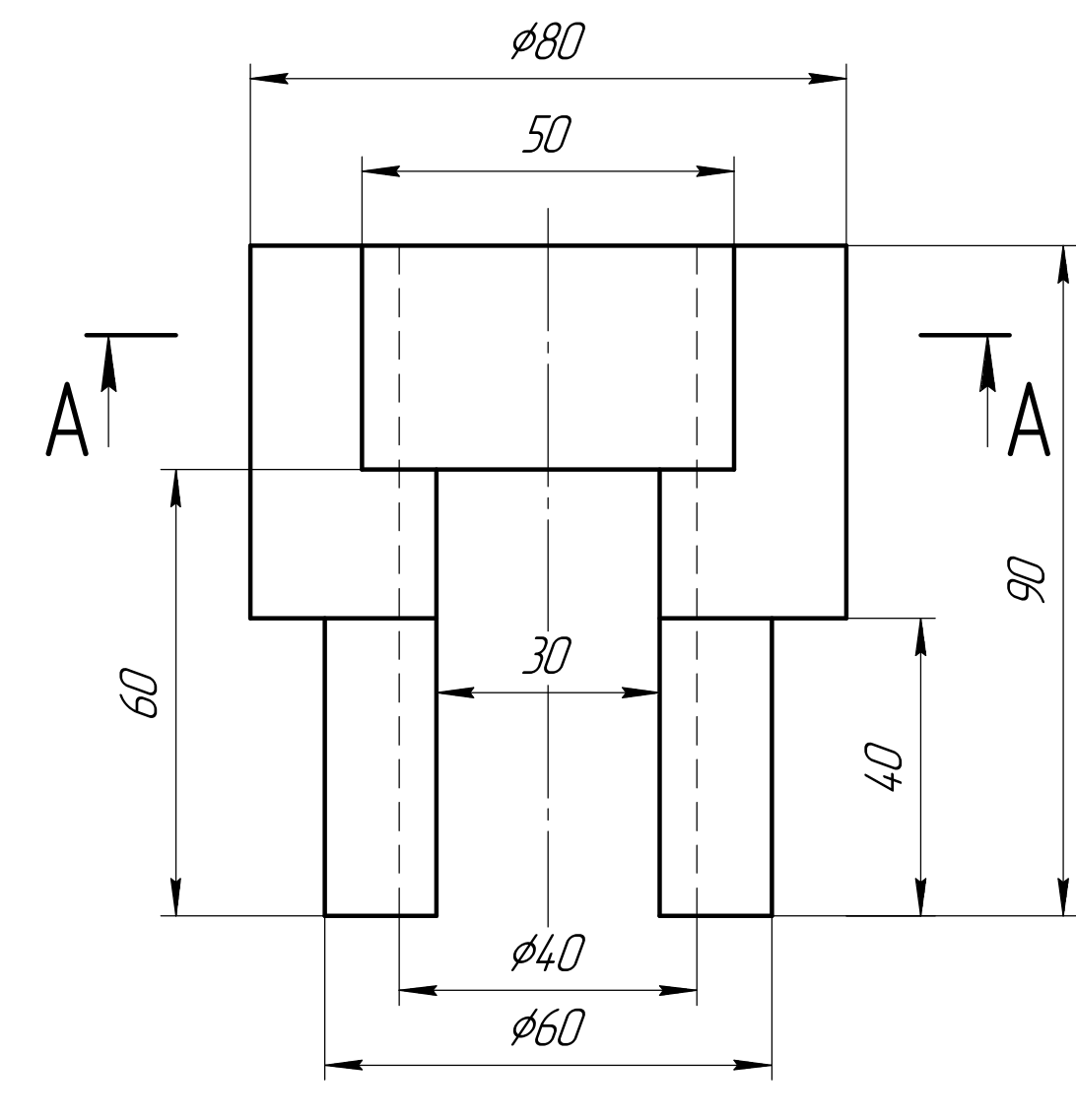
вариант 15 Вид спереди
